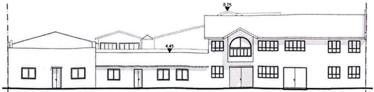
Figura 3. Elevación principal frente fachada continua.
